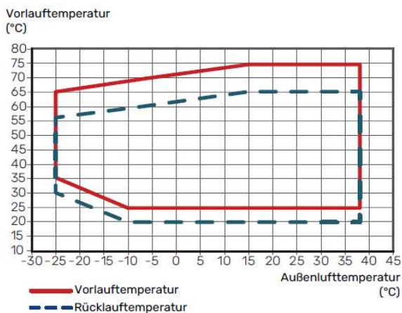
S2125-8 Betriebsbereich Heizung
